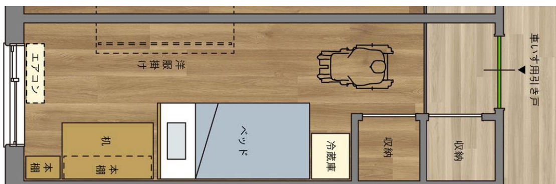
○居室間取り
