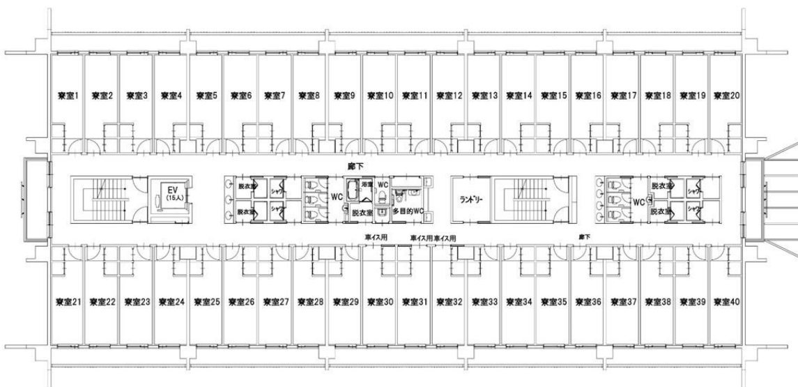
○居室間取り
